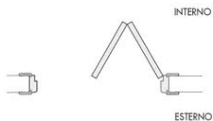
PIEGHEVOLE LIBRO SPINGERE DESTRA
